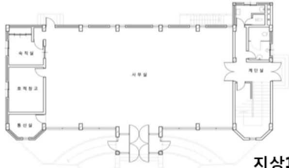
지상2층 평면도
