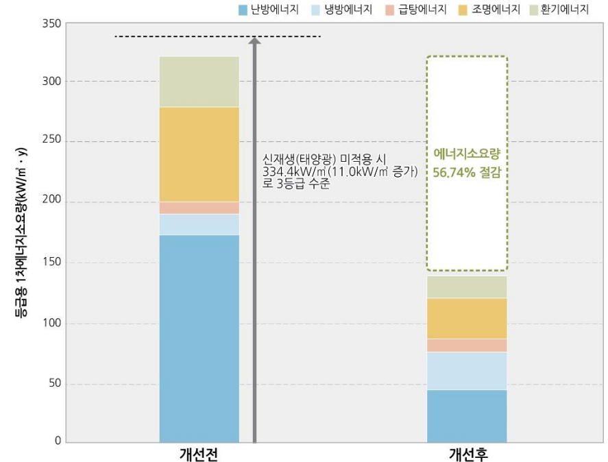
에너지 시뮬레이션을 통한 절감효과 확인
